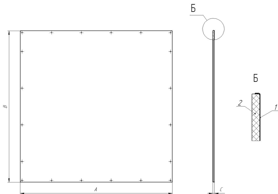
Рисунок 1 — Общий вид экрана для защиты стен
